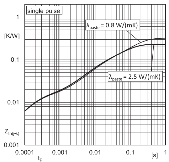
Fig. 2: Typ. transient thermal impedance
